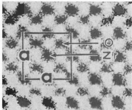
▲○は酸素、Zrはジルコニウムの各原子、aは隣り合うZr 同士の間隔(1億分の5.2cm)
